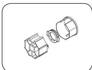
Kit Rueda/Corona Motor M40 - Tubo Octogonal 40 (COD. MOMAKIT001)
